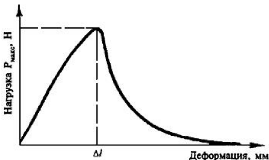
Рисунок 1. Запись диаграммы "нагрузка-деформация"
