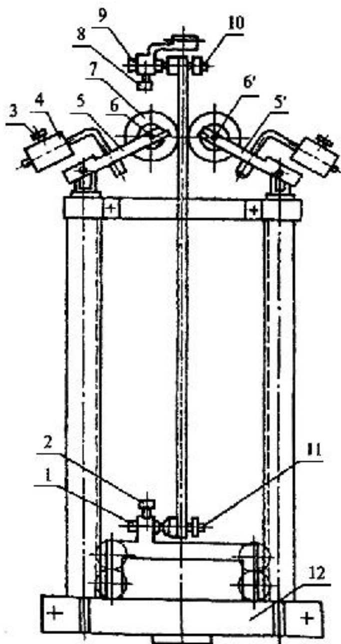
Рисунок 7. Приспособление для определения липкости
